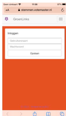
Afb. 1: inlogscherm
